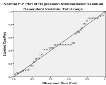
Gambar 2. Uji Normalitas
