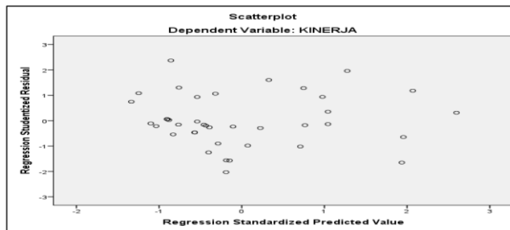
Gambar 3. Sebaran variansi data
